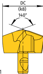
Геометрия U для сталей и нержавеющих сталей
