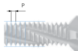
Резьбофрезерование: шаг резьбы P определяется программой ЧПУ (обработка по винтовой интерполяции).
