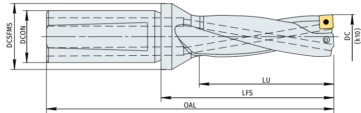
Хвостовик WHISTLE NOTCH с фланцем
