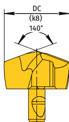
Геометрия U для сталей и нержавеющей сталей
