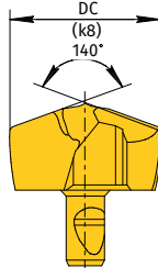
Геометрия K для чугунов
