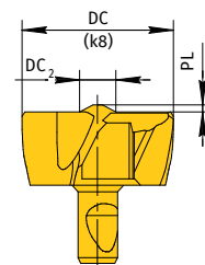
Геометрия C универсального применения, для цекования
