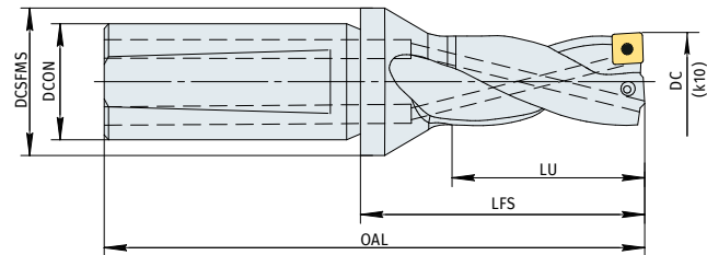
Хвостовик WHISTLE NOTCH с фланцем
