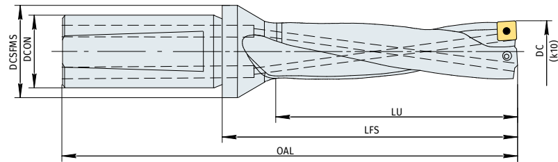
Хвостовик WHISTLE NOTCH с фланцем
