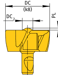
Геометрия C универсального применения, для цекования
