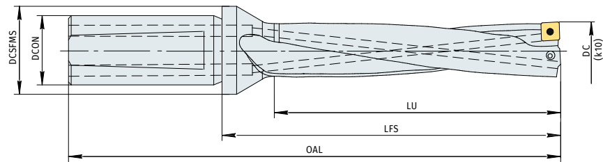
Хвостовик WHISTLE NOTCH с фланцем
