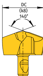
Геометрия K для чугунов
